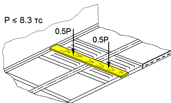
Рисунок 10 – Размещение подкладок на одном люке полувагона
